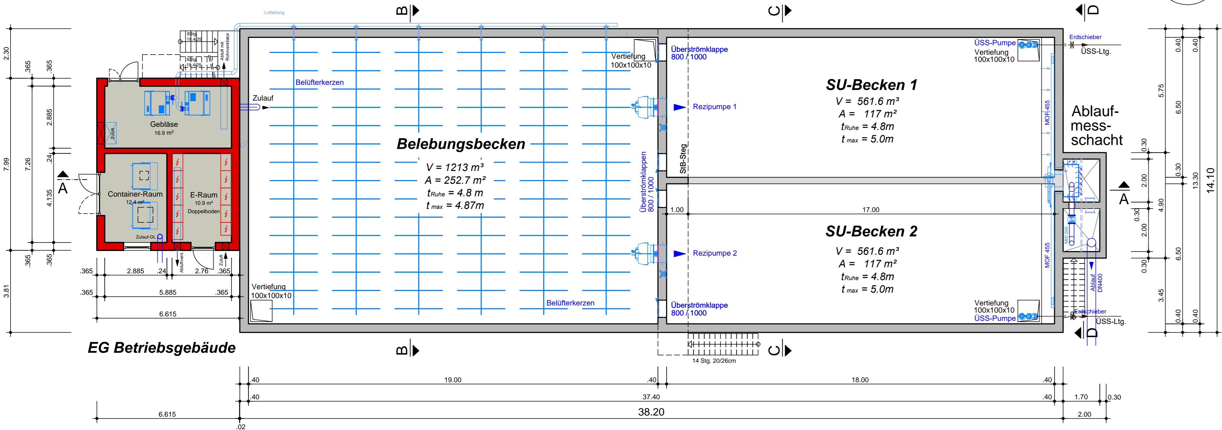
EG Betriebsgebäude / Grundriss BIOCOS-Becken
