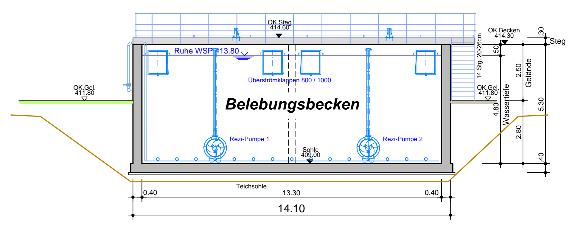
Schnitt C-C
